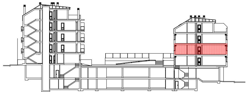
SECCION
